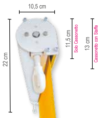
Cassonetto 7000 R
