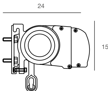
Scivolo Braccio Newbox
