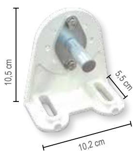
Staffa
