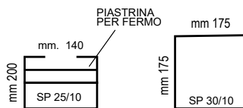
TRAVE PERIMETRALE
