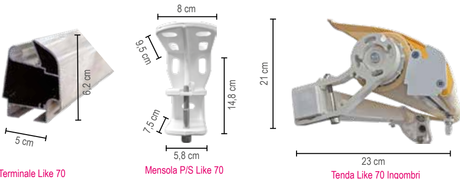
Tenda Like 70 Ingombri
