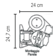
Ingombri Rodi
