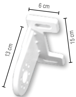
Staffa Parete / Soffitto 6000 IN
