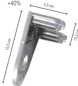
Staffa a tenda Classica
