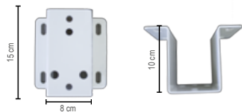
Distanziale opzionale a richiesta € 22,00 cad.
