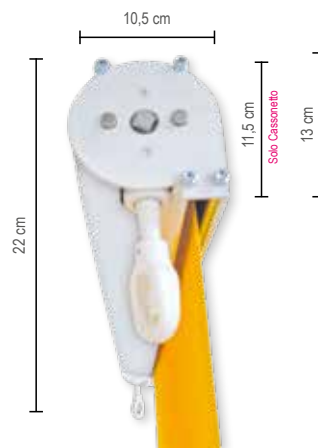
Cassonetto 4000 R
