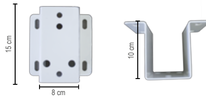
Distanziale opzionale a richiesta € 22,00 cad.
