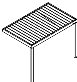
Montaggio addossata lame perpendicolari alla parete
